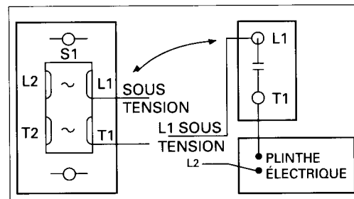
Figure 2.2 Installation d'un condensateur dans un thermostat typique
