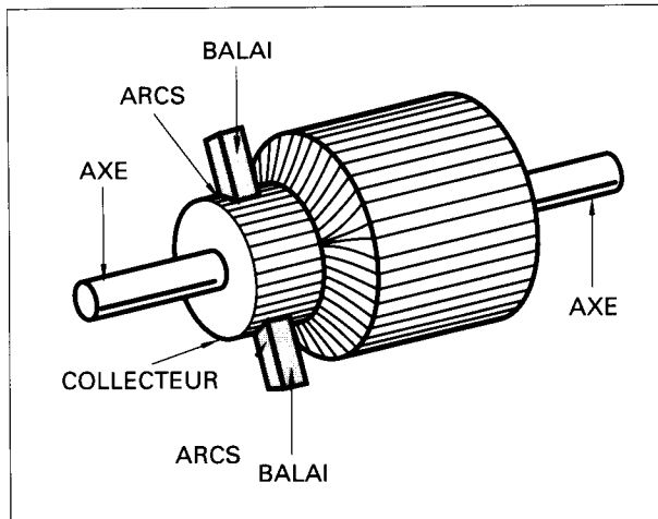
Figure 2.7 Vue de côté d'une armature typique; des arcs (étincelles) sont produits entre le collecteur et chaque balai
