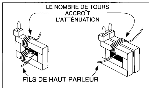
Figure 1.7 Fils de haut-parleur non blindés enroulés autour d'un noyau en ferrite
