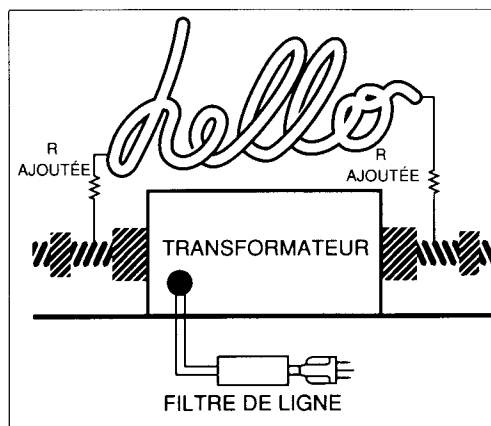
Figure 2.6 Installation d'un filtre de ligne dans le transformateur d'une lampe au néon et de résistances de 10 kohms en série avec chaque fil sous haute tension
