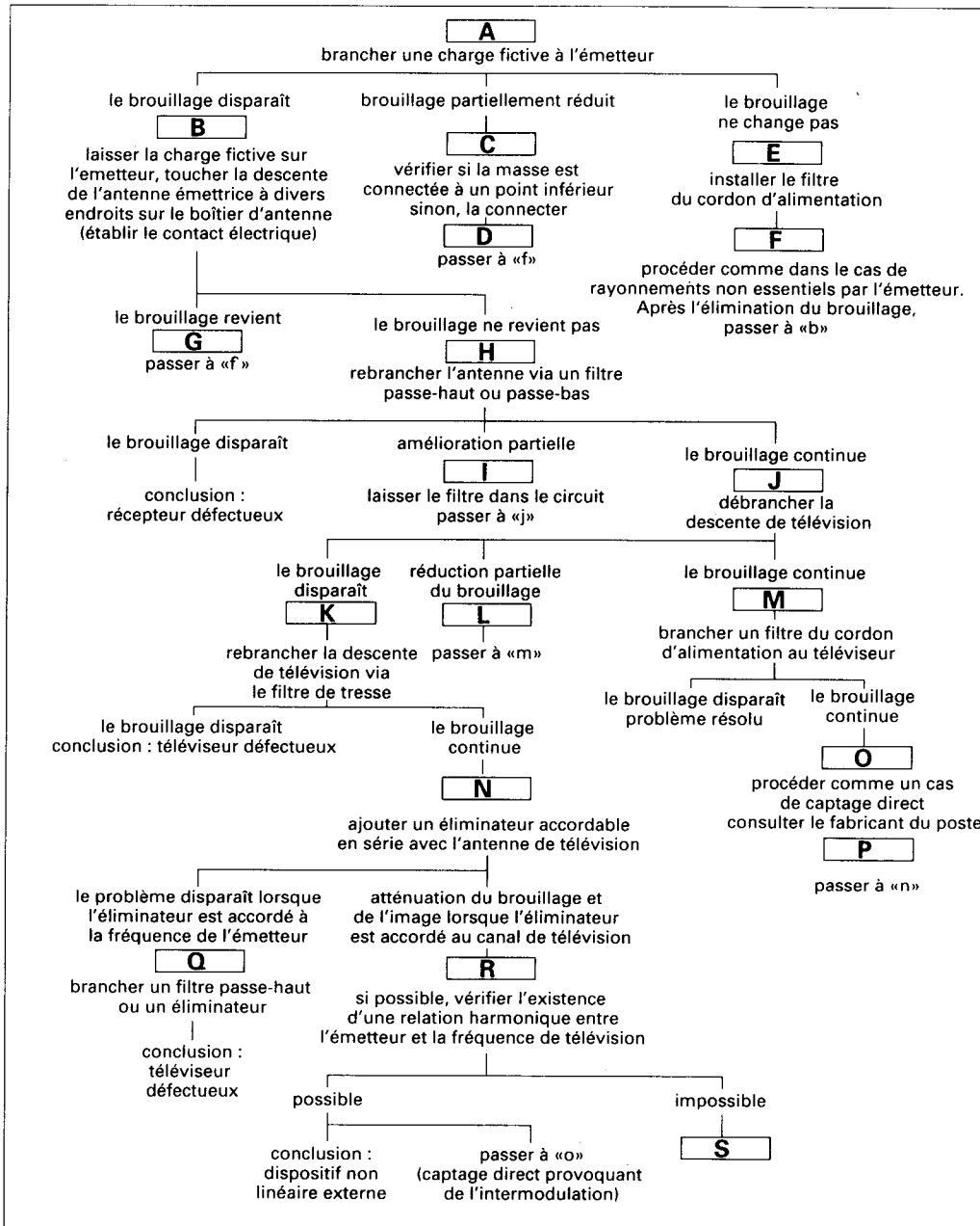
Figure 3.1 Guide pour localiser le brouillage par un émetteur
