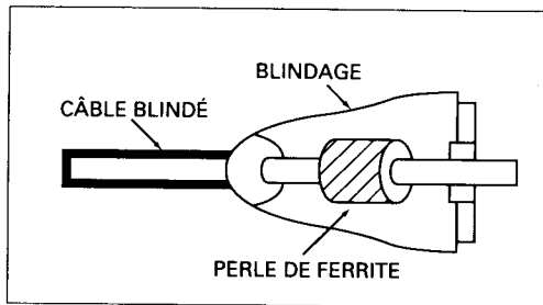
Figure 1.9 Montage d'une perle de ferrite sur un fil de haut-parleur
