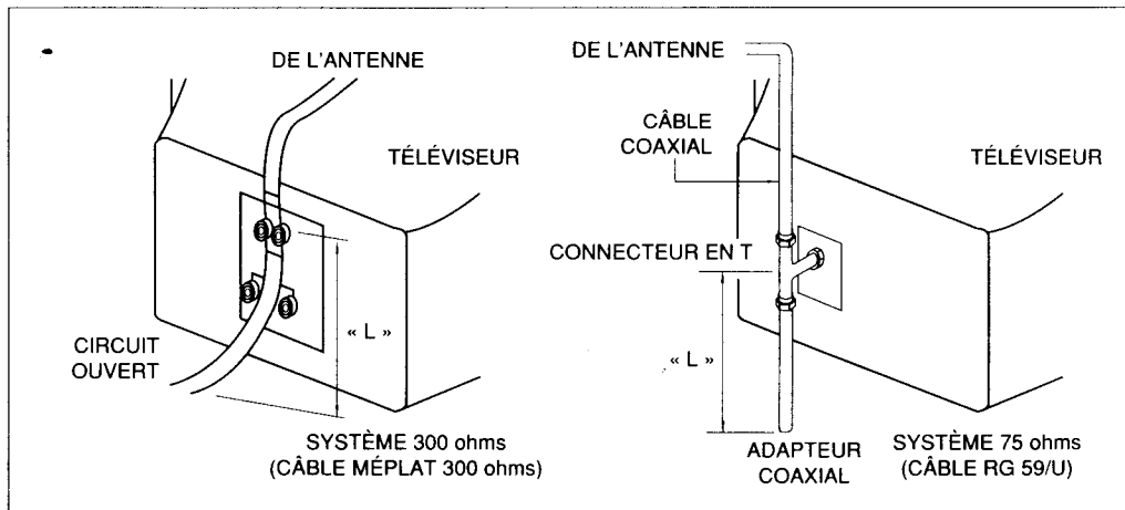
Figure 3.12 Utilisation de bras de réactance quart d'onde pour éliminer le brouillage
