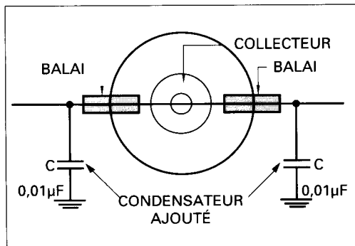
Figure 2.8 Vue de l'extrémité d'une armature de moteur montrant l'emplacement des condensateurs
