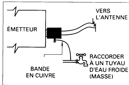
Figure 3.5 Procédure pour une bonne mise à la terre
