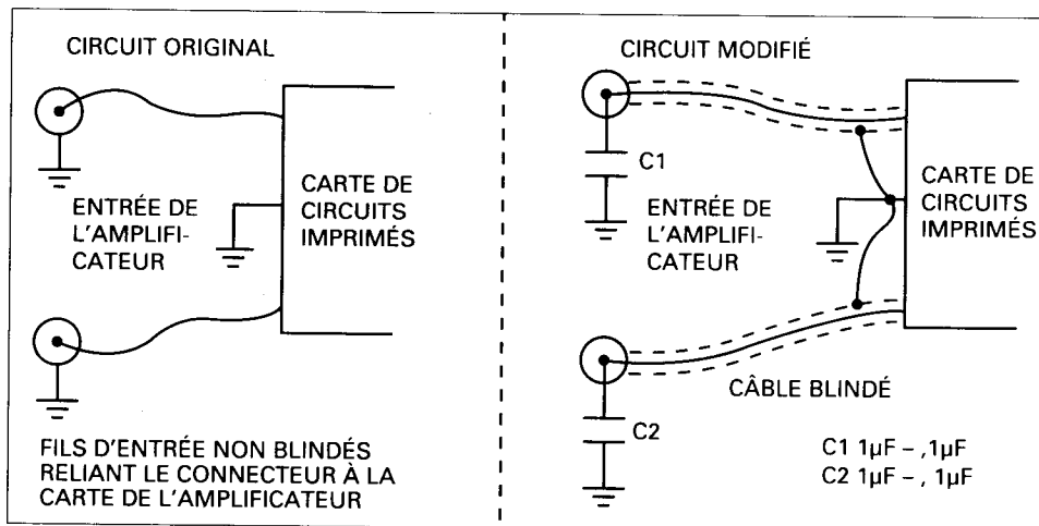
Figure 1.10 Installation d'un fil blindé entre le connecteur d'entrée de l'amplificateur et la carte de circuits imprimés
