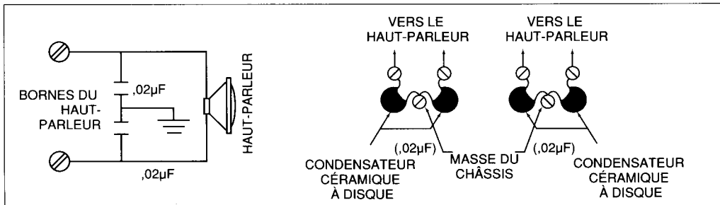
Figure 1.8 Dérivation des fils de haut-parleur
