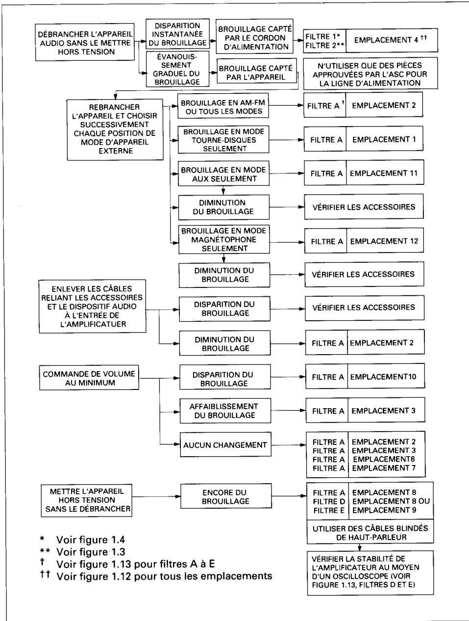
Figure 1.11 Table de dépannage des problèmes de brouillage de radiofréquence dans une chaîne stéréophonique (partie 1)
