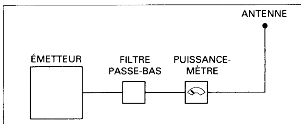
Figure 3.7 Installation d'un filtre passe-bas dans une descente d'antenne
