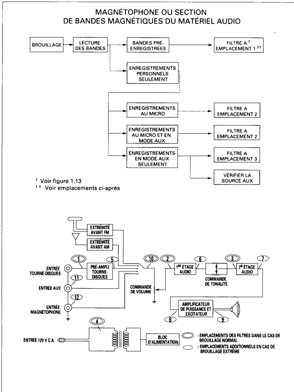
Figure 1.12 Table de dépannage des problèmes de brouillage de radiofréquence dans une chaîne stéréophonique (partie 2)
