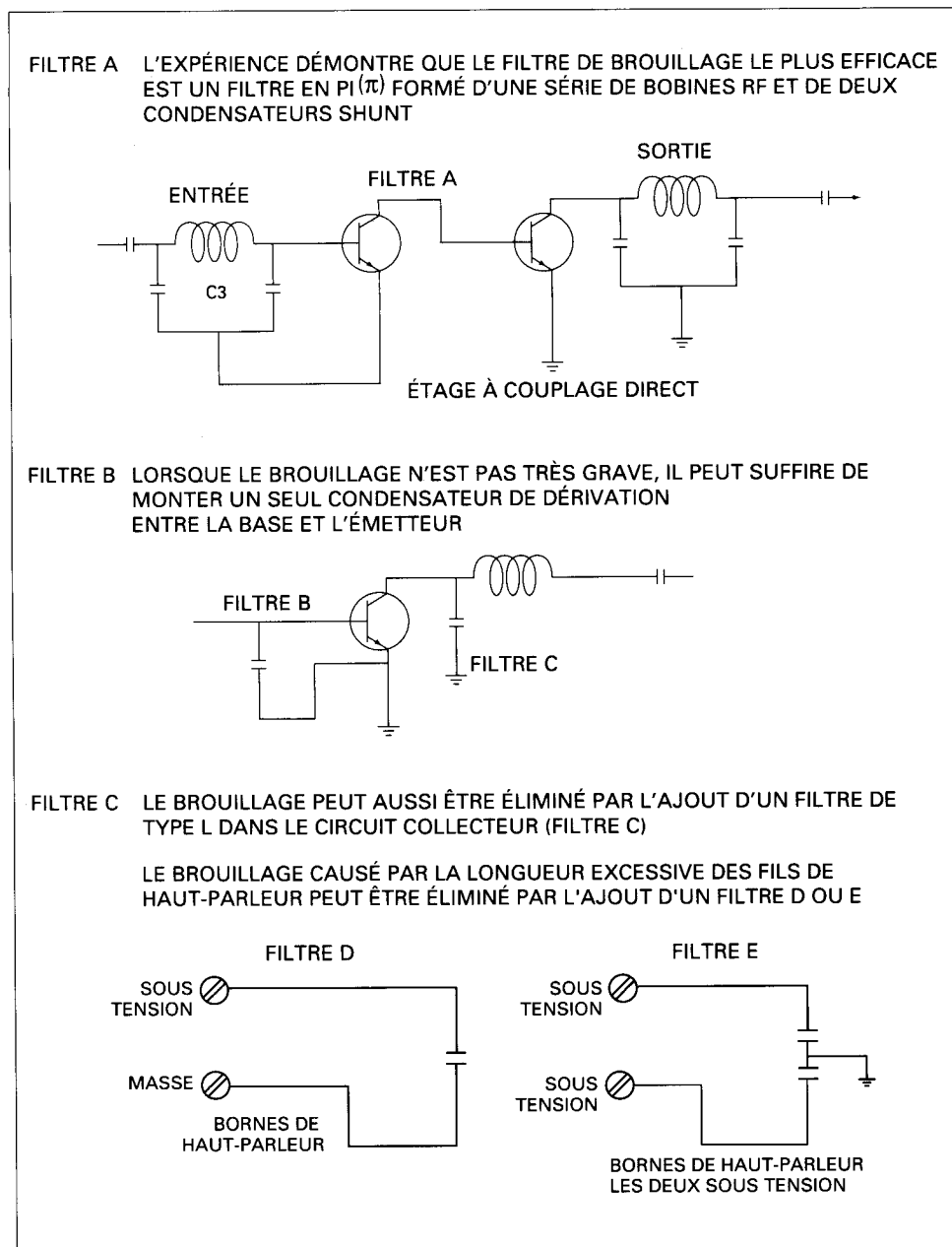
Figure 1.13 Installation d'un condensateur entre la base et l'émetteur et aux bornes de haut-parleur
