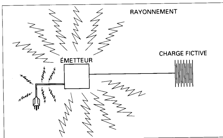
Figure 3.6 Fonctionnement d'un émetteur avec une charge fictive blindée
