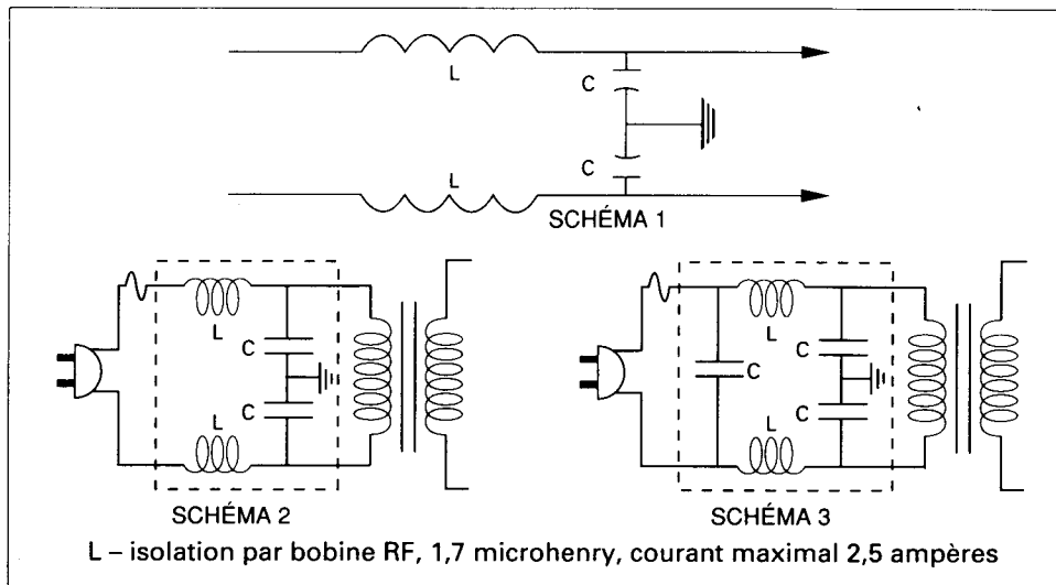
Figure 1.4 Trois schémas de filtre c.a.
