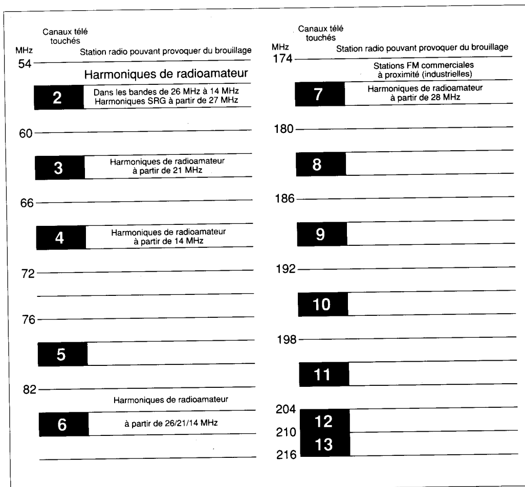
Figure 3.2 Relations entre les canaux de télévision VHF et les stations radio qui peuvent produire du brouillage
