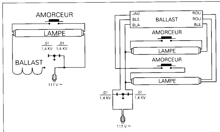
Figure 2.5 Installation de condensateurs dans des lampes fluorescentes
