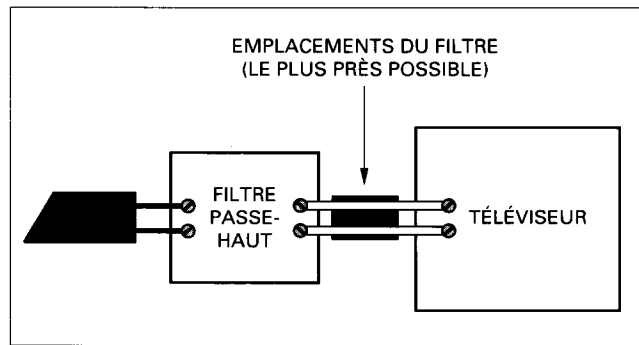
Figure 3.10 Installation d'un filtre passe-haut aux entrées d'antenne du téléviseur
