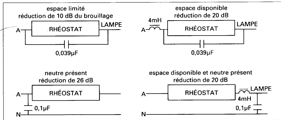
Figure 2.4 Quatre emplacements possibles pour la suppression du brouillage dû à un rhéostat d'éclairage
