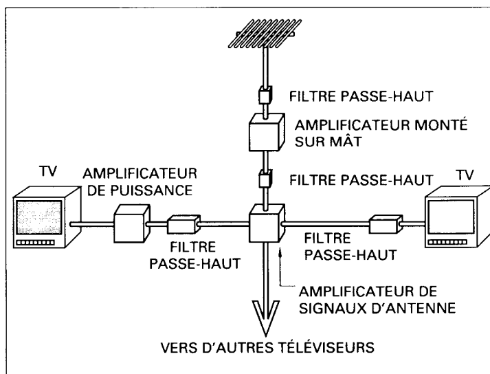
Figure 3.8 Installation de filtres passe-haut dans les systèmes d'antennes
