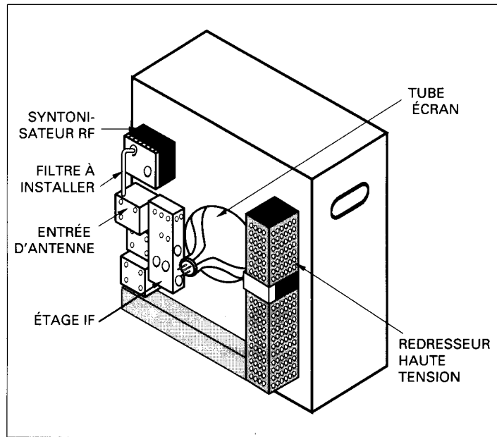
Figure 3.9 Installation d'un filtre passe-haut dans un téléviseur
