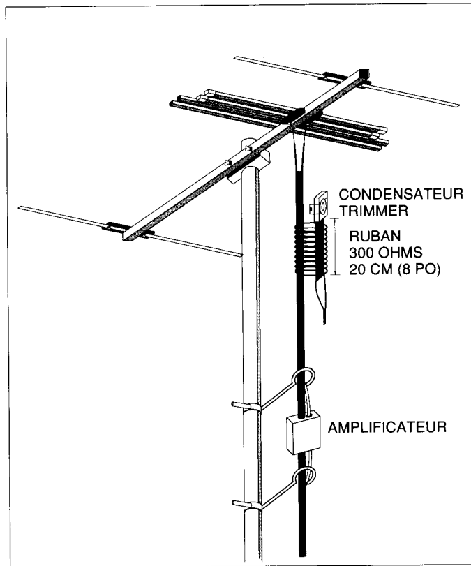
Figure 3.13 Installation d'un éliminateur accordable en le fixant sur la descente d'antenne avec le ruban 300 ohms
