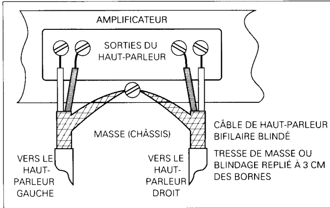
Figure 1.6 Méthode de connexion des fils blindés de haut-parleur, avec la méthode de mise à la masse de la tresse de blindage
