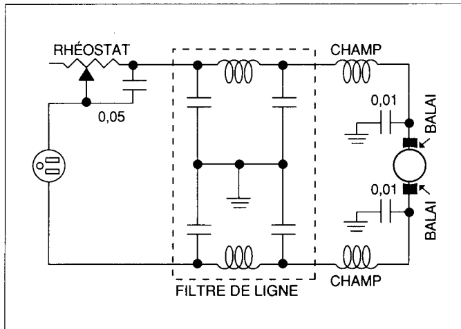
Figure 2.9 Suppression du brouillage produit par une machine à coudre
