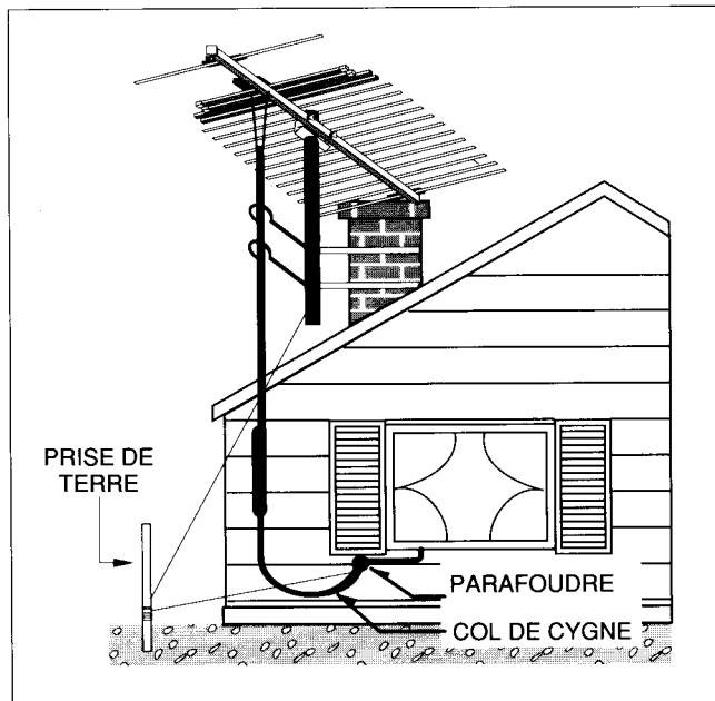
Figure 4.1 Installation de l'antenne avec parafoudre
