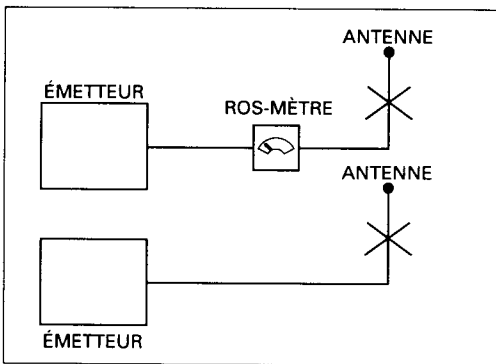
Figure 3.4 Mesure du rapport d'ondes stationnaires au moyen d'un ROS-mètre
