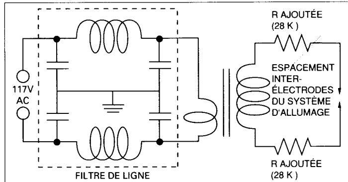
Figure 2.3 Suppression du brouillage dans les systèmes d'allumage de la plupart des fournaies à l'huile ou au gaz modernes
